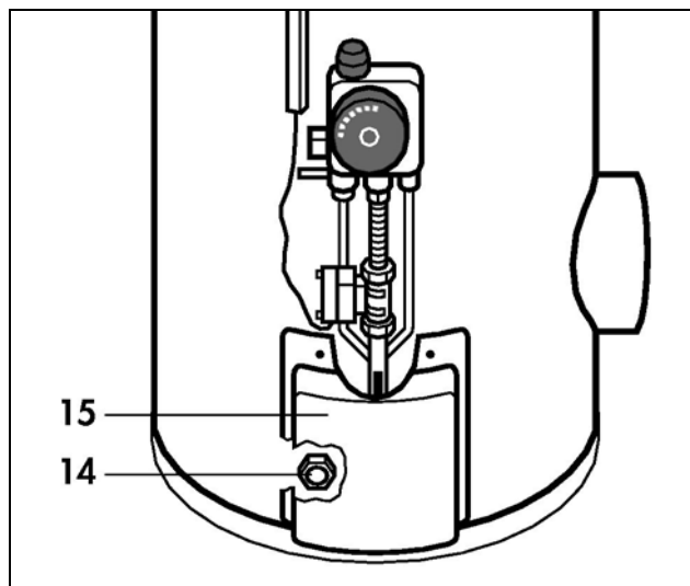
Рис. 5 Слив воды из аппарата atmoSTOR VGH
