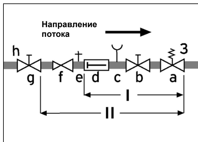
Рис. 11 Предохранительные группы
